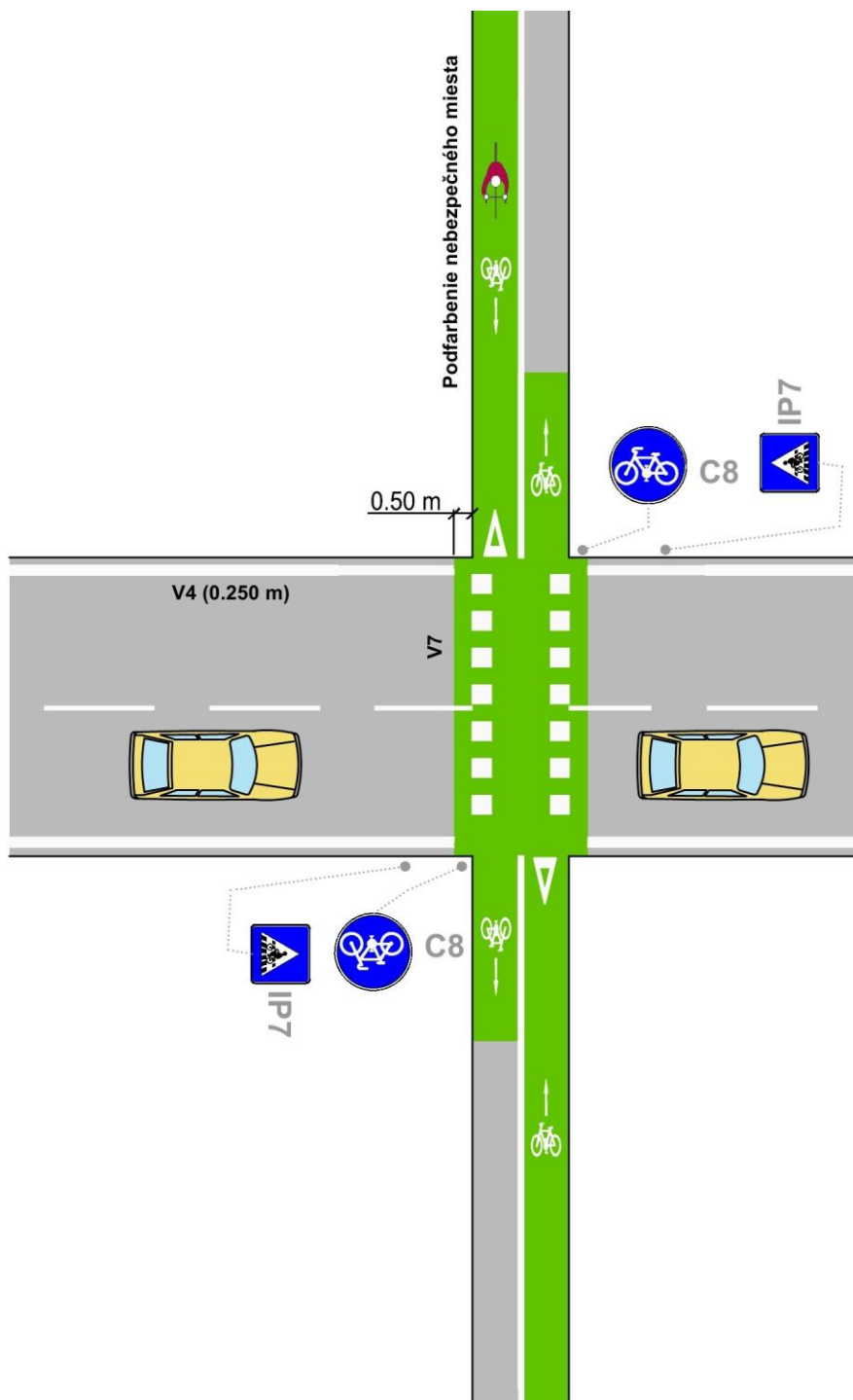
Obrázok 80 Priechod pre cyklistov – podfarbený
