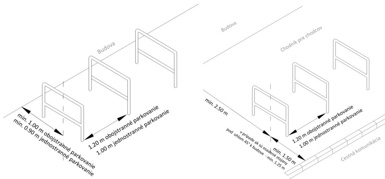
Obrázok 38 Pričné umiestnenie stojanov na bicykle pri budove
