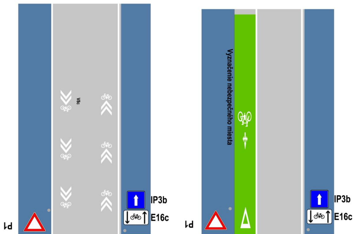
Obrázok 97 Ukončenie CYK na jednosmerných komunikáciách
