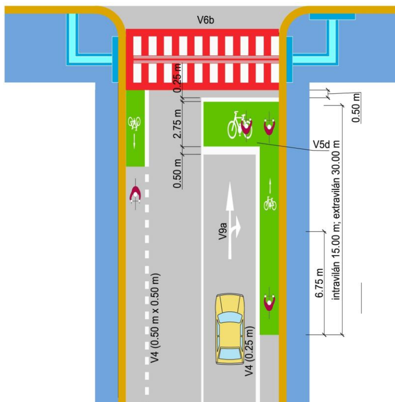
Obrázok 76 Rozmery priestoru pre cyklistov s bočným cyklopruhom
