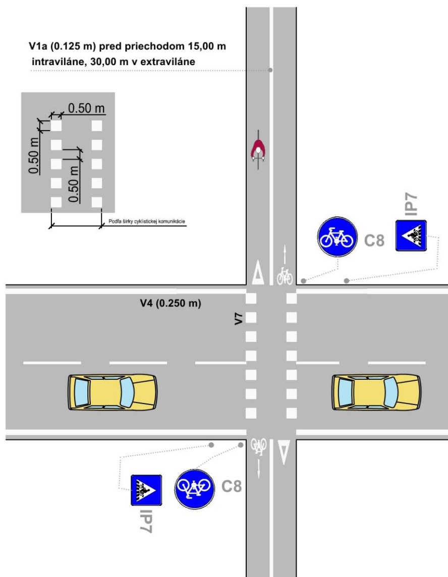
Obrázok 79 Priechod pre cyklistov
