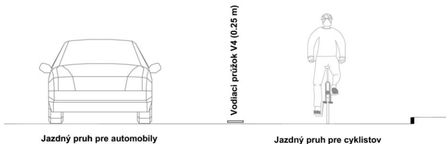
Obrázok 5 Oddelenie cyklistického pruhu a jazdného pruhu. Využíva sa na mestských komunikáciách typu B2, B3, C1 až C3, D1 a D2 a na cestách II. a III. triedy.
