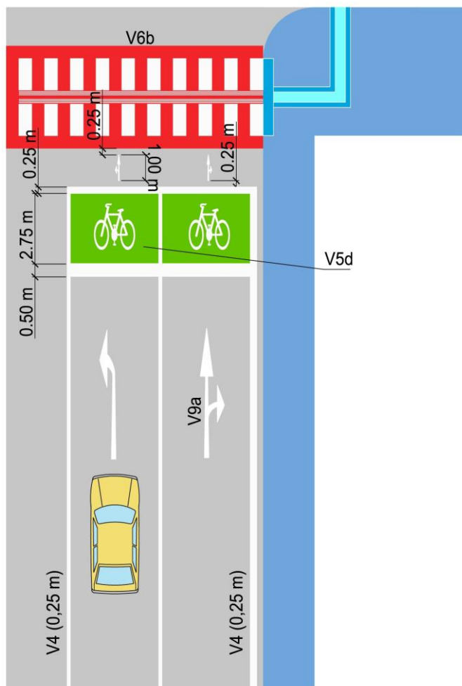
Obrázok 77 Rozmery priestoru pre cyklistov so smerovými šípkami pre cyklistov
