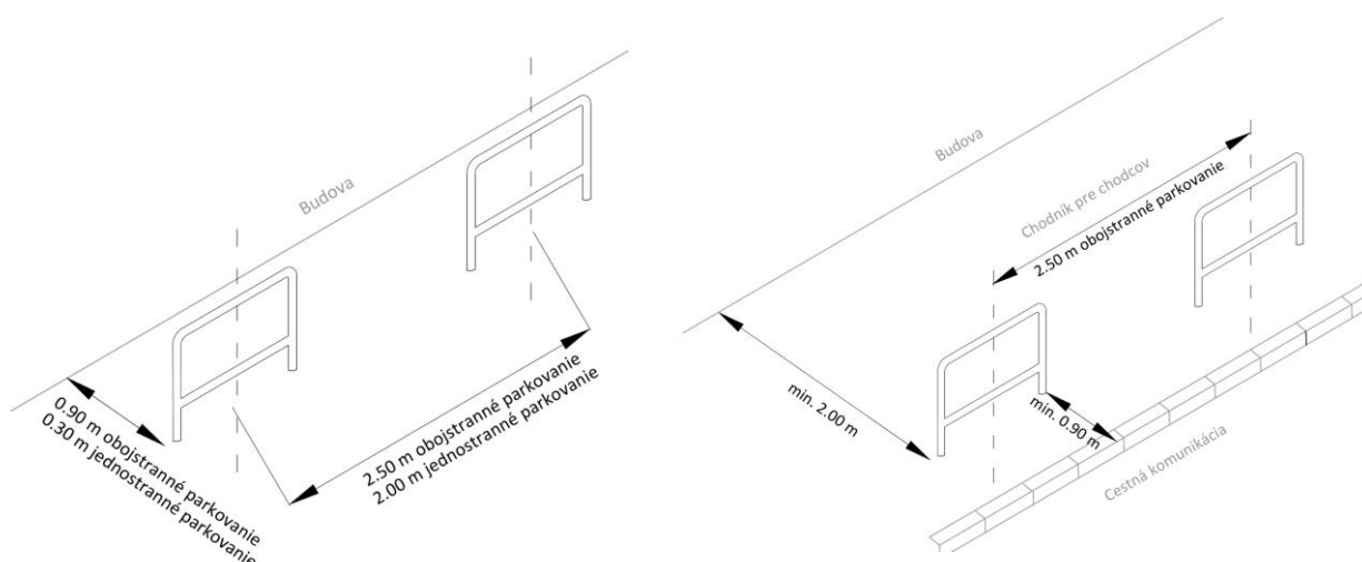
Obrázok 36 Pozdĺžne umiestnenie stojanov na bicykle pri budove
