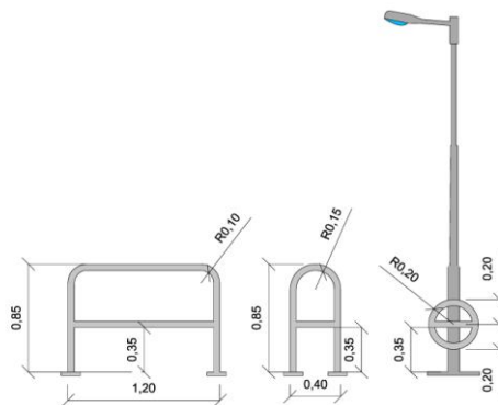
Obrázok 35 Príklady rozmerov cyklistických stojanov
