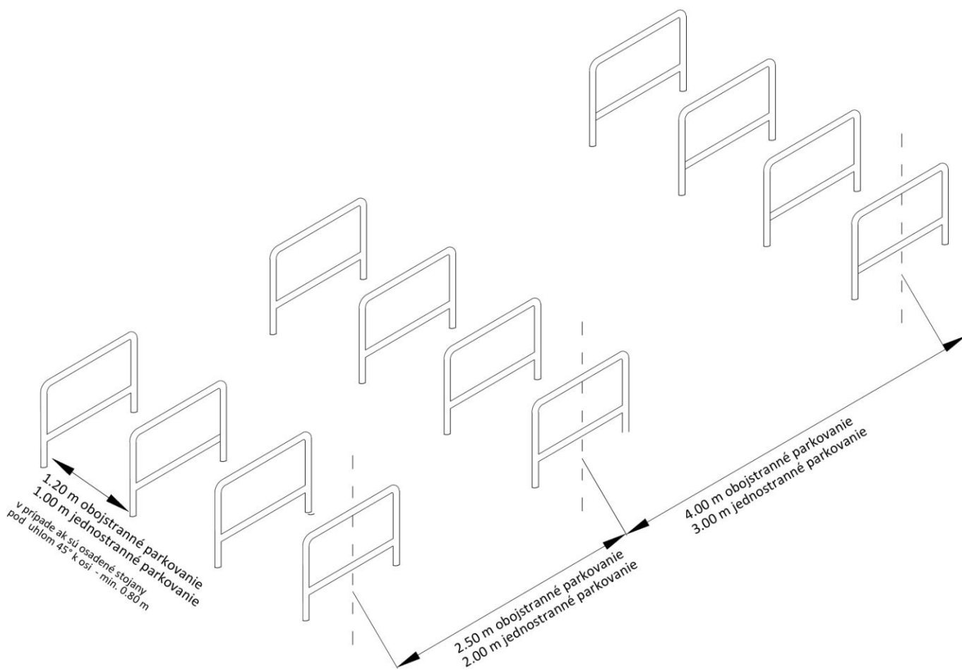
Obrázok 40 Umiestnenie stojanov na odstavňových plochách
