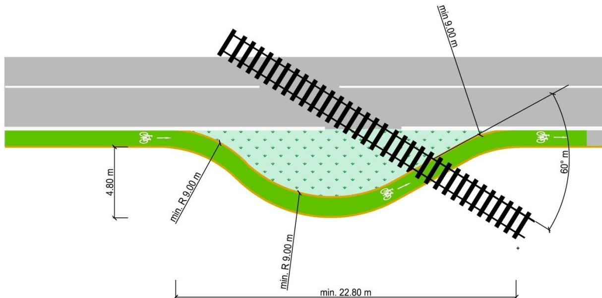
Obrázok 105 Prejazd cez koľajovú trať odsunutím cyklistického pruhu
