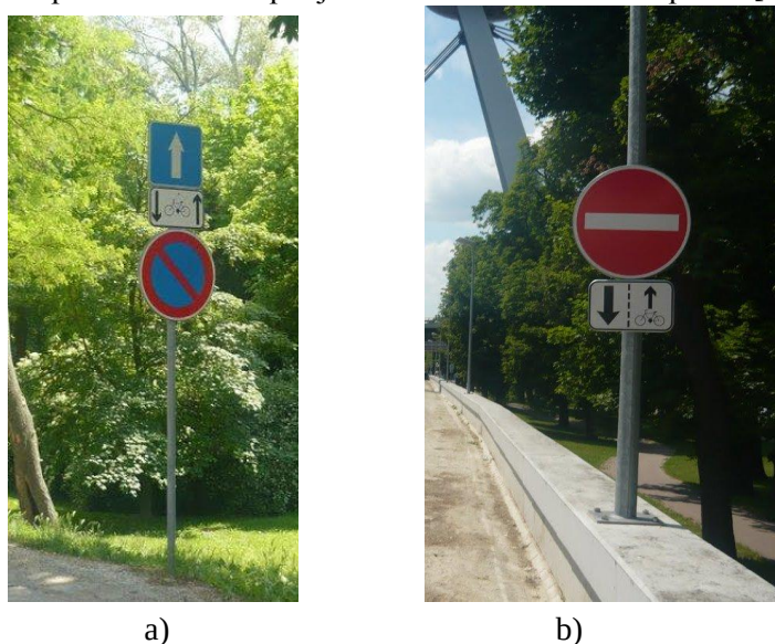
Obrázok 61 Dopravné značenie pre jednosmerné komunikácie podľa [Z1]
