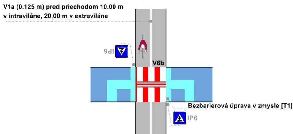
Obrázok 102 Križovanie pomocou priechodu pre chodcov s podfarbením
