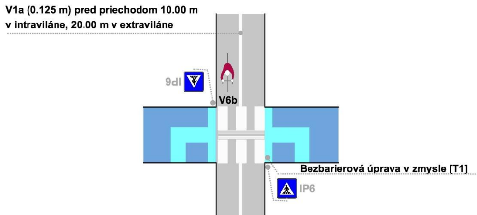
Obrázok 101 Križovanie pomocou priechodu pre chodcov bez podfarbenia
