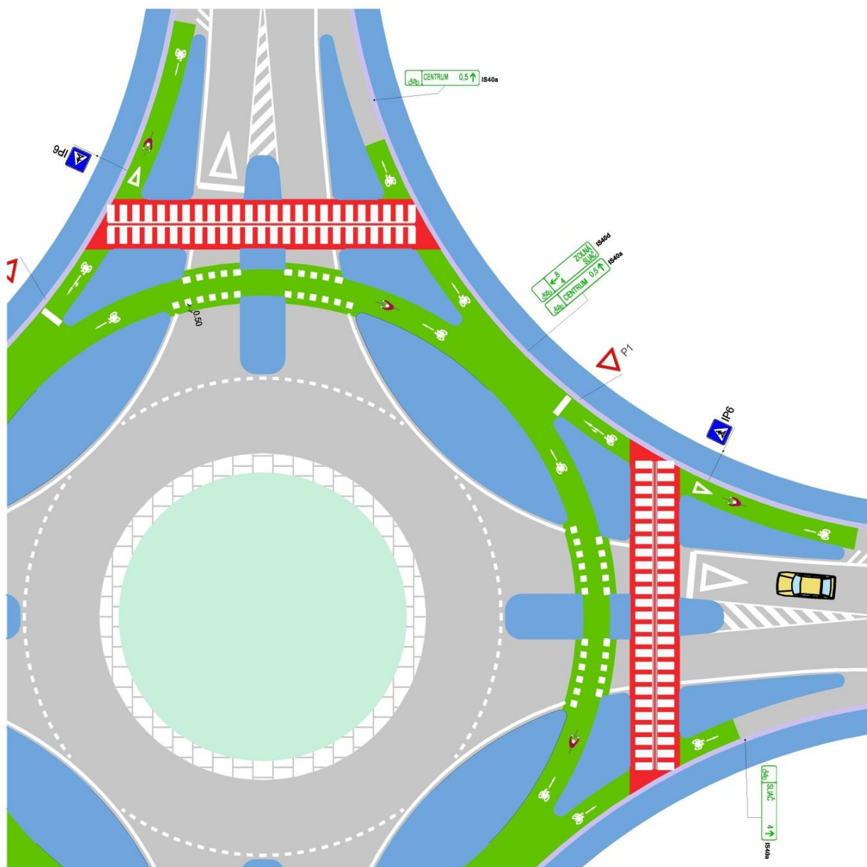
Obrázok 115 Okružná križovatka s okružným vedením cyklistov
