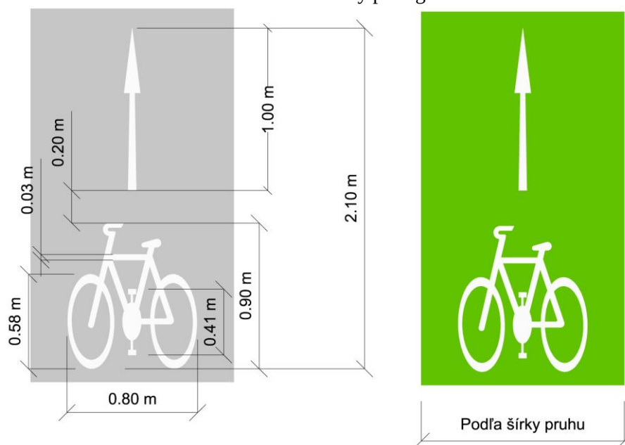
Obrázok 74 Rozmery piktogramu so smerovou šípkou
