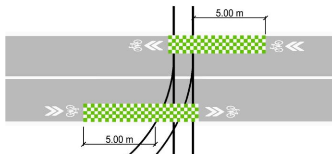
Obrázok 108 Prejazd koridoru pre cyklistov cez električkovú trať pomocou dopravného značenia
