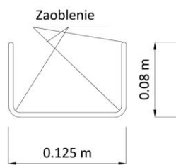
Obrázok 45 rozmery cyklistického žliabku
