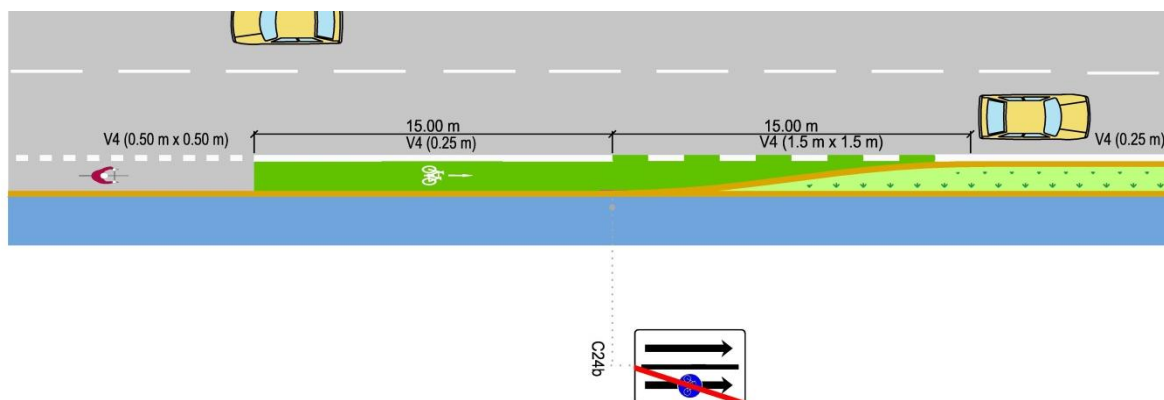
Obrázok 16 Ukončenie cyklistického pruhu
