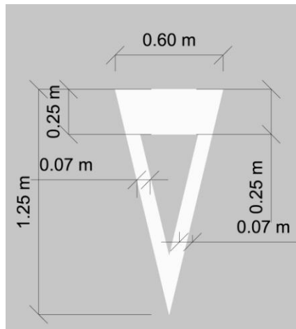
Obrázok 75 Rozmery cyklistického trojuholníka
