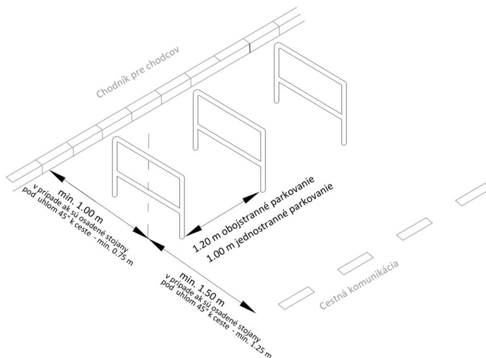
Obrázok 42 Umiestnenie stojanov na PK
