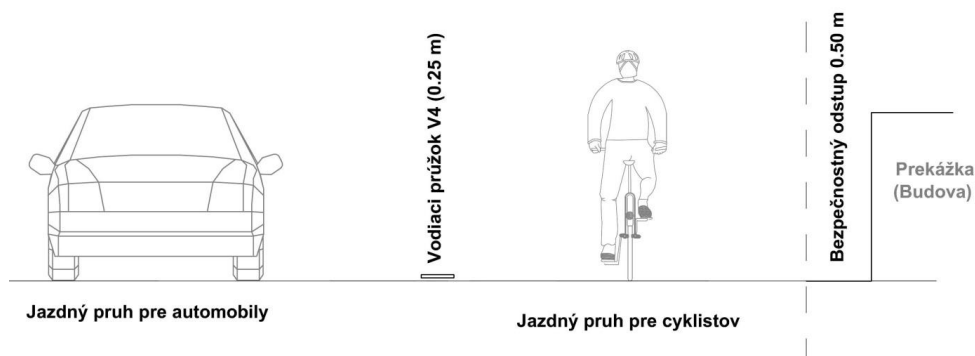
Obrázok 7 Oddelenie cyklistického pruhu a jazdného pruhu s bezpečnostným odstupom 0,50 m od prekážky.
