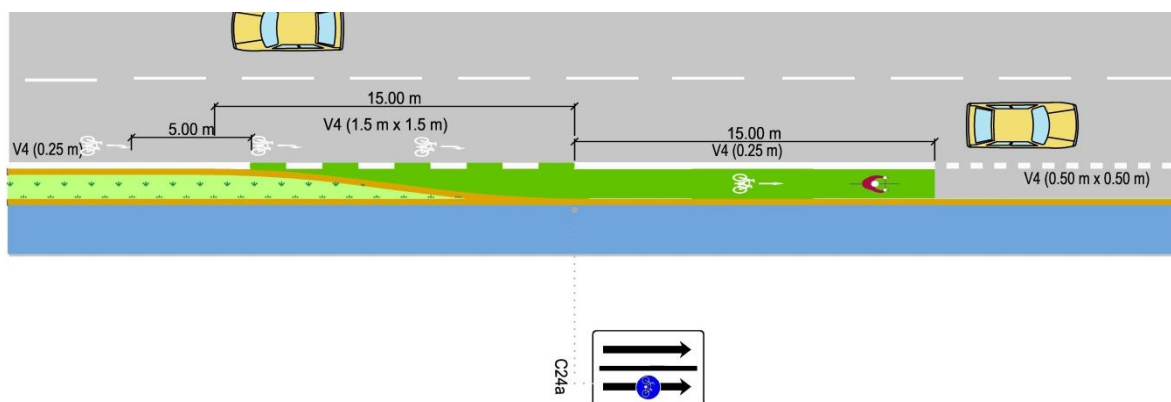
Obrázok 15 Začiatok cyklistického pruhu
