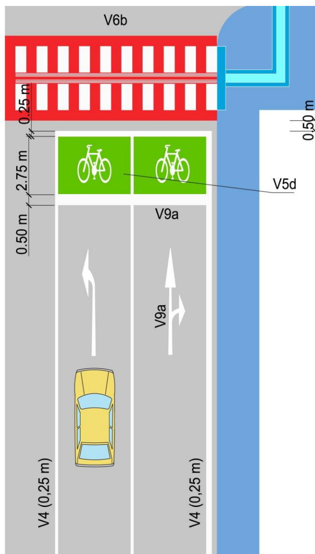
Obrázok 78 Rozmery priestoru pre cyklistov bez bočného cyklopruhu
