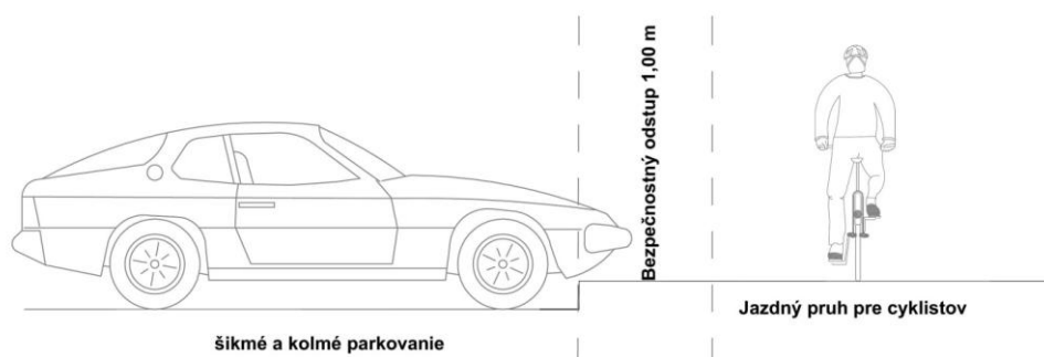
Obrázok 11 Cyklistický pruh vľavo pri šikmom a kolmom parkovaní
