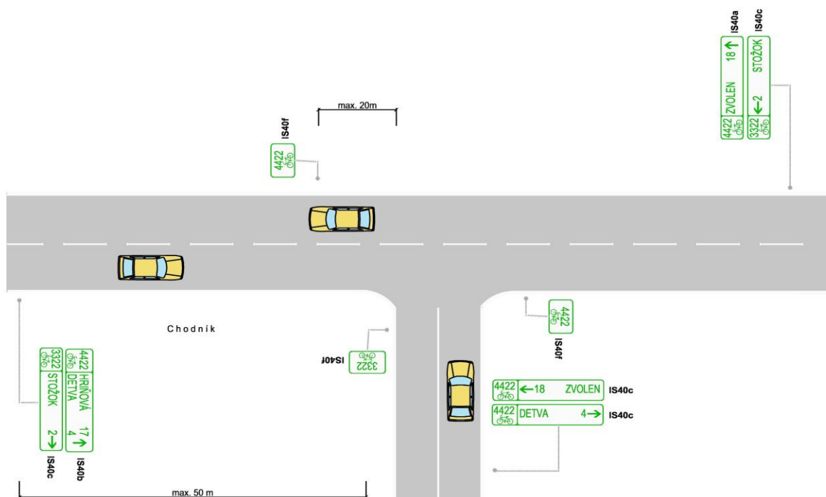
Obrázok 71 Príklad umiestnenia smerového dopravného značenia
