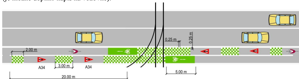
Obrázok 107 Prejazd CYK cez električkovú trať pomocou dopravného značenia
