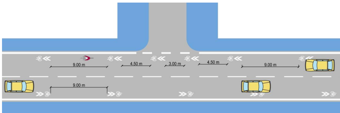
Obrázok 34 Prevedenie koridoru pre cyklistov cez križovatku
