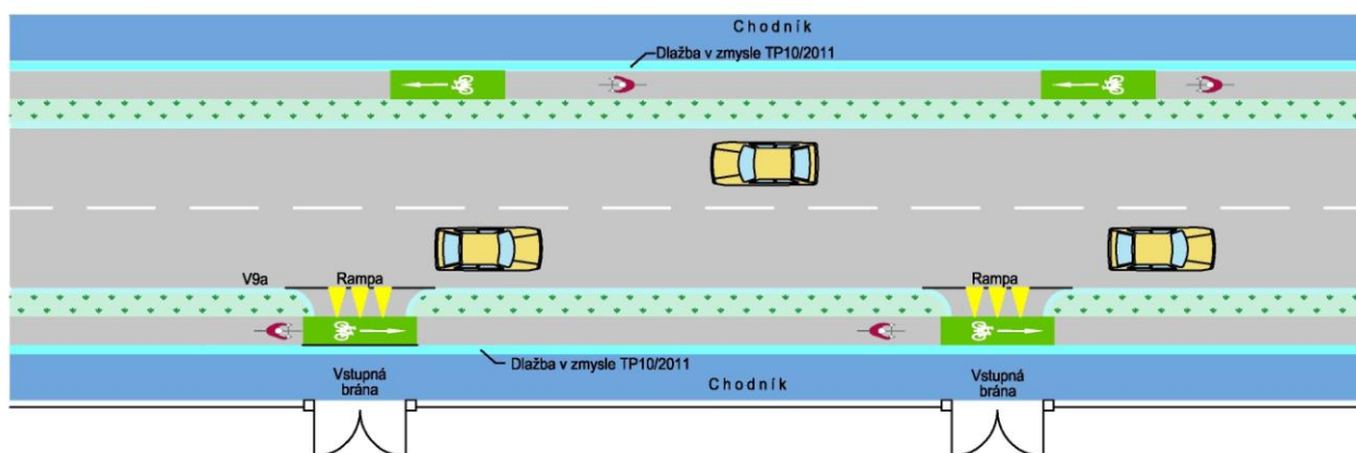
Obrázok 98 Príklad prejazdu cyklistického pruhu cez vjazdy
