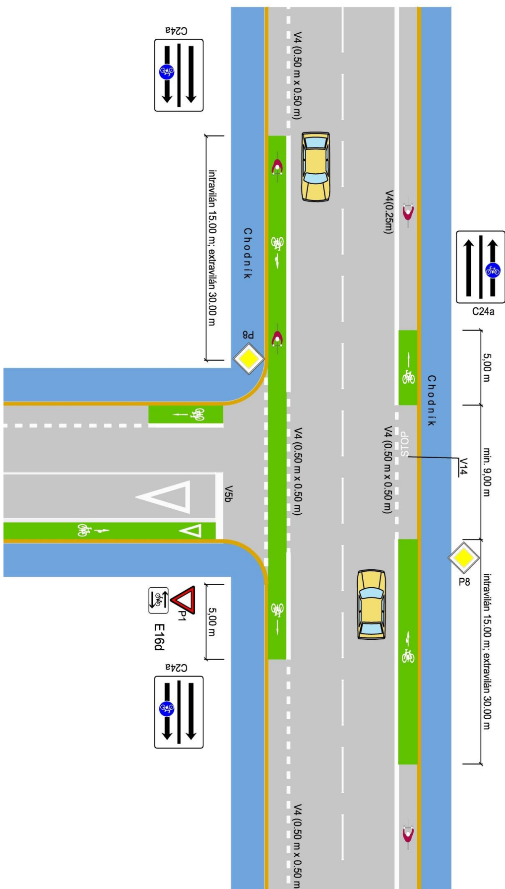
Obrázok 110 Styková križovatka s cyklistickými pruhmi na hlavnej a vedľajšej komunikácii
