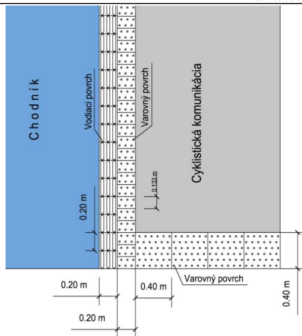
Obrázok 27 Dlažba pri oddelení chodcov a cyklistov
