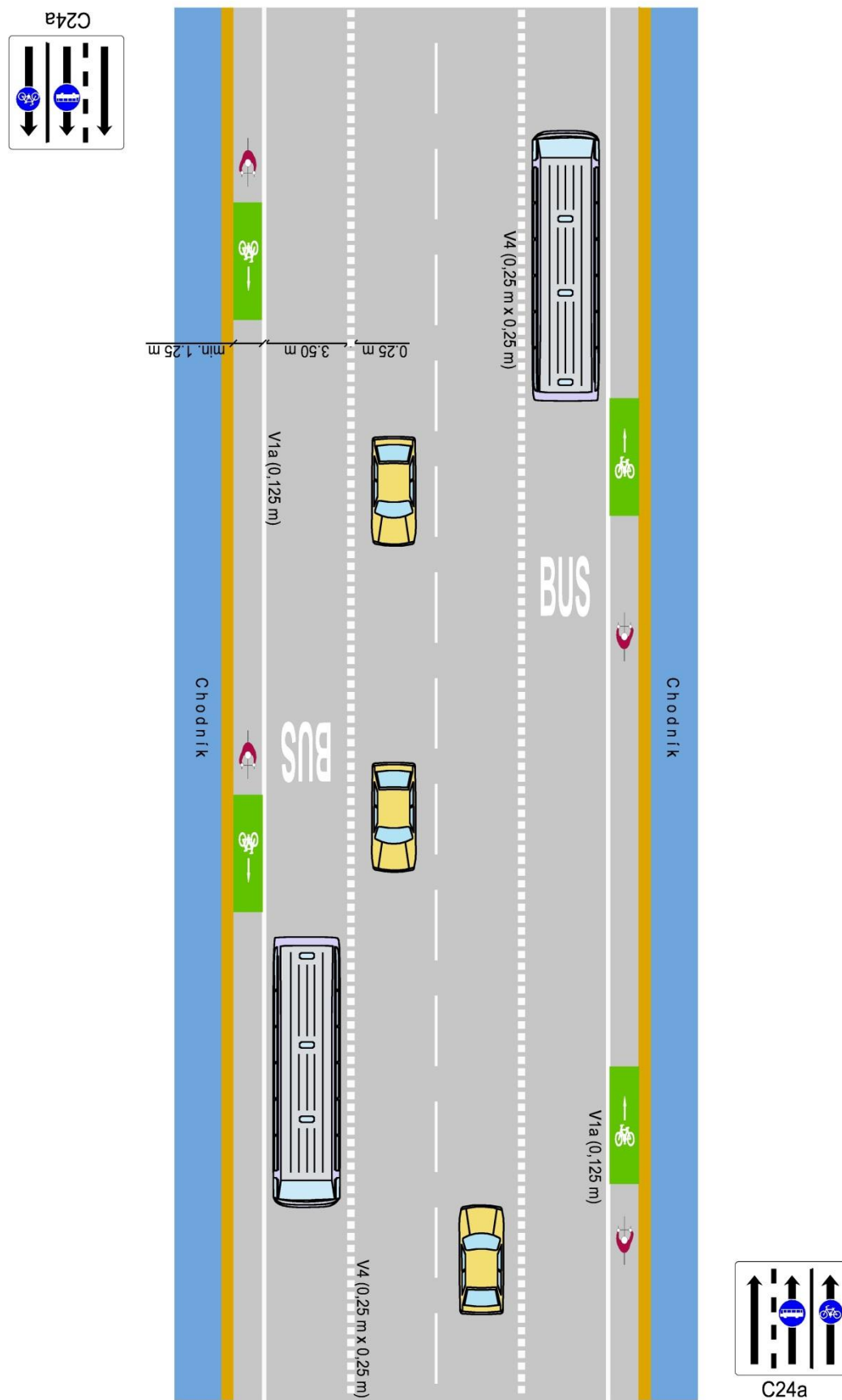
Obrázok 91 Samostatný pruh pre cyklistov a autobusy
