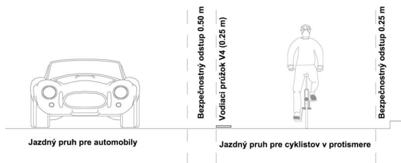
Obrázok 14 Protismerný cyklistický pruh
