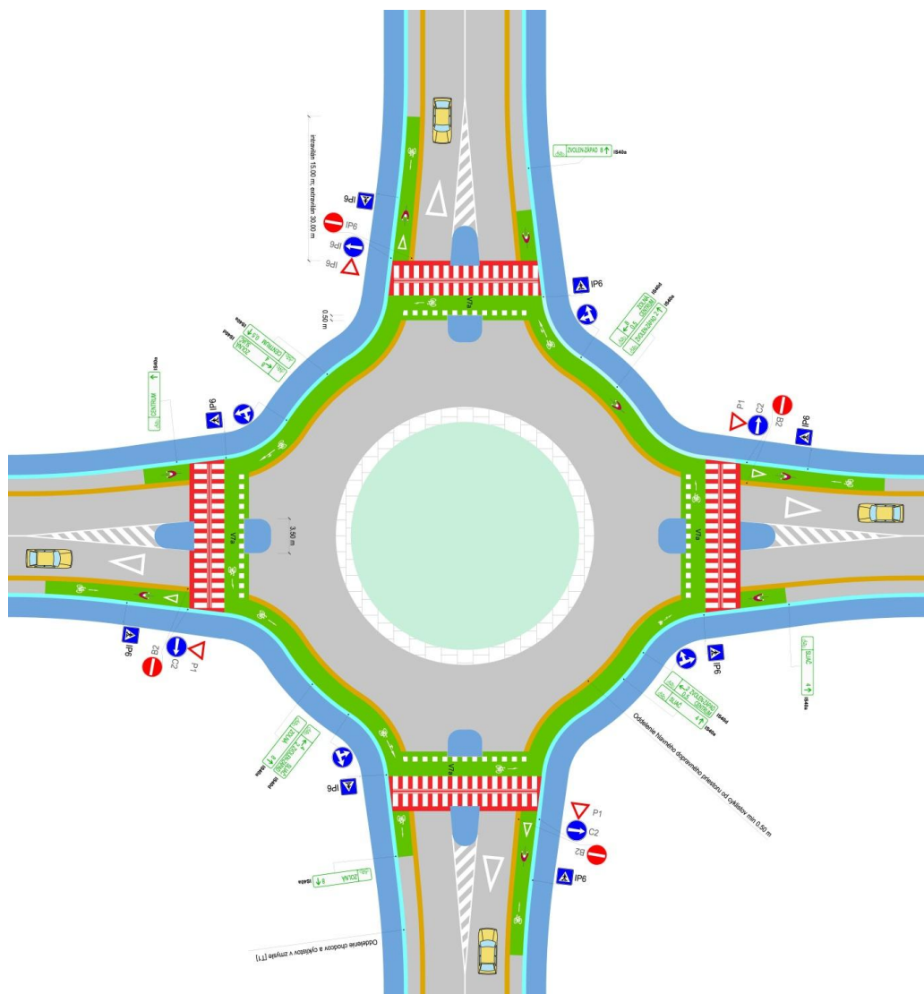
Obrázok 114 Okružná križovatka
