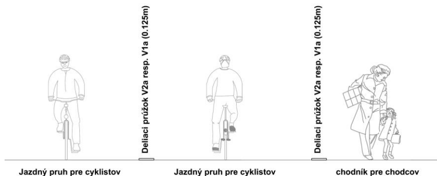
Obrázok 30 Oddelenie chodcov a cyklistov pomocou deliaceho prúžku
