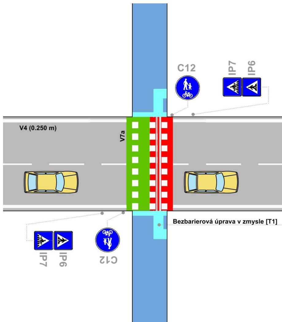
Obrázok 81 Spoločný priechod pre cyklistov a chodcov
