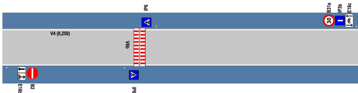
Obrázok 93 Povolenie jazdy cyklistom do jednosmernej komunikácie
