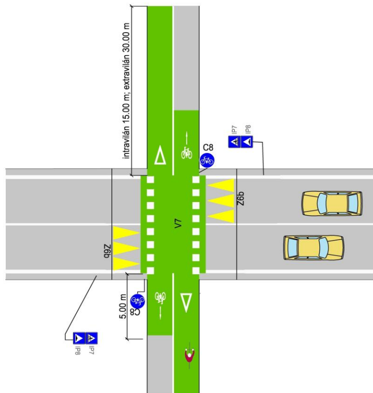
Obrázok 99 Zvýšený priechod pre cyklistov
