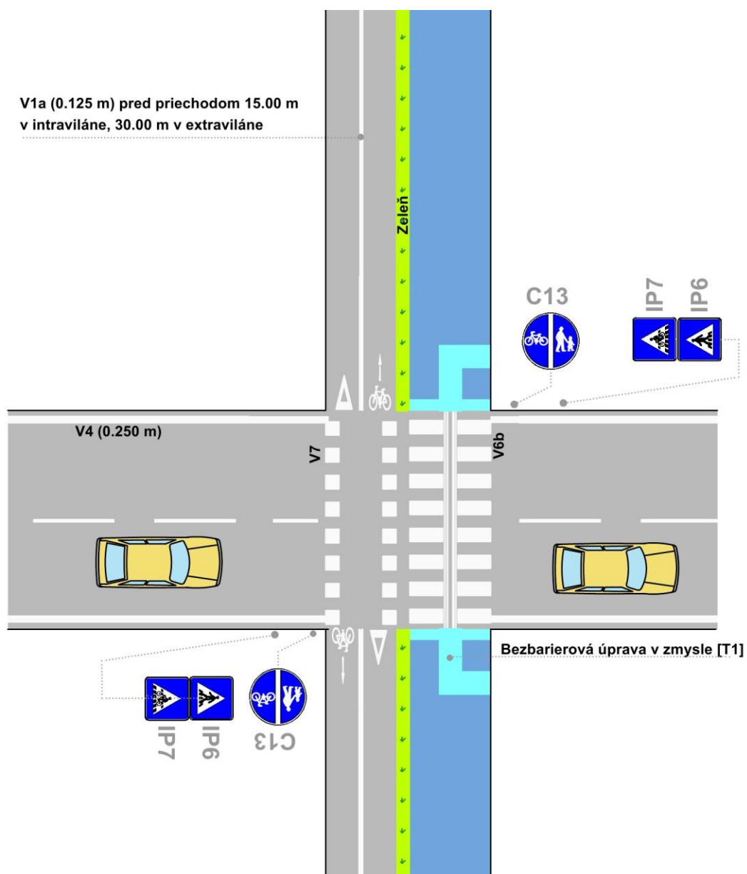
Obrázok 84 Nepodfarbený priechod pre cyklistov vedľa priechodu pre chodcov
