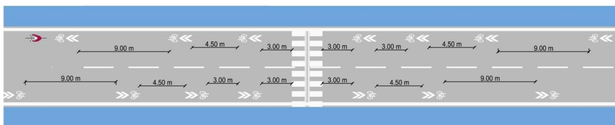
Obrázok 33 Prevedenie koridoru pre cyklistov cez priechod pre chodcov
