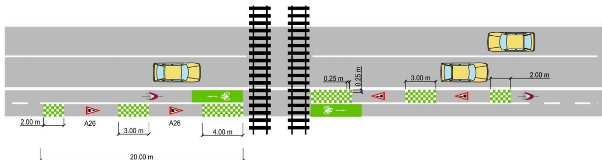
Obrázok 106 Prejazd CYK cez železničnú trať pomocou dopravného značenia
