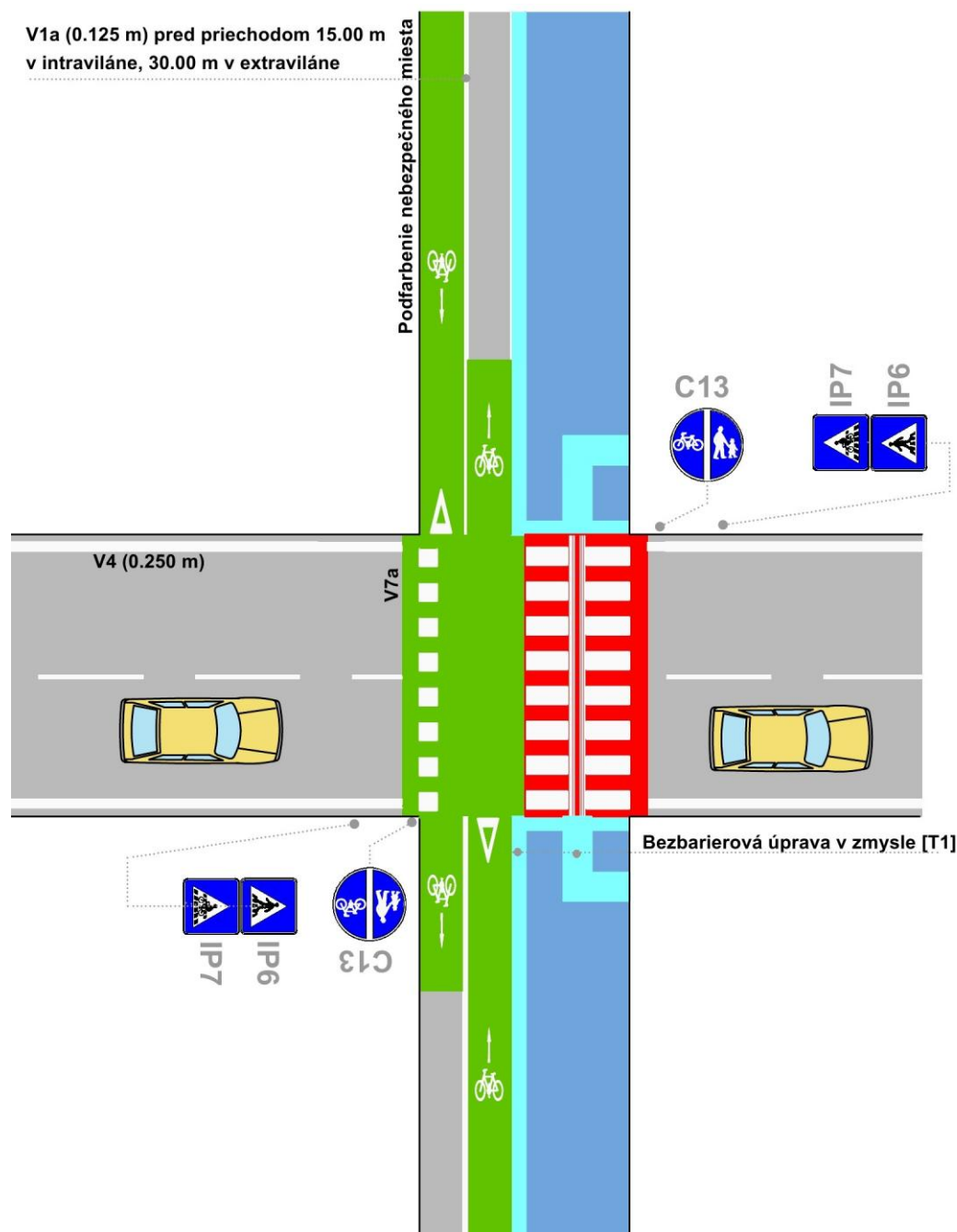
Obrázok 83 Podfarbený priechod pre cyklistov primknutý k priechodu pre chodcov
