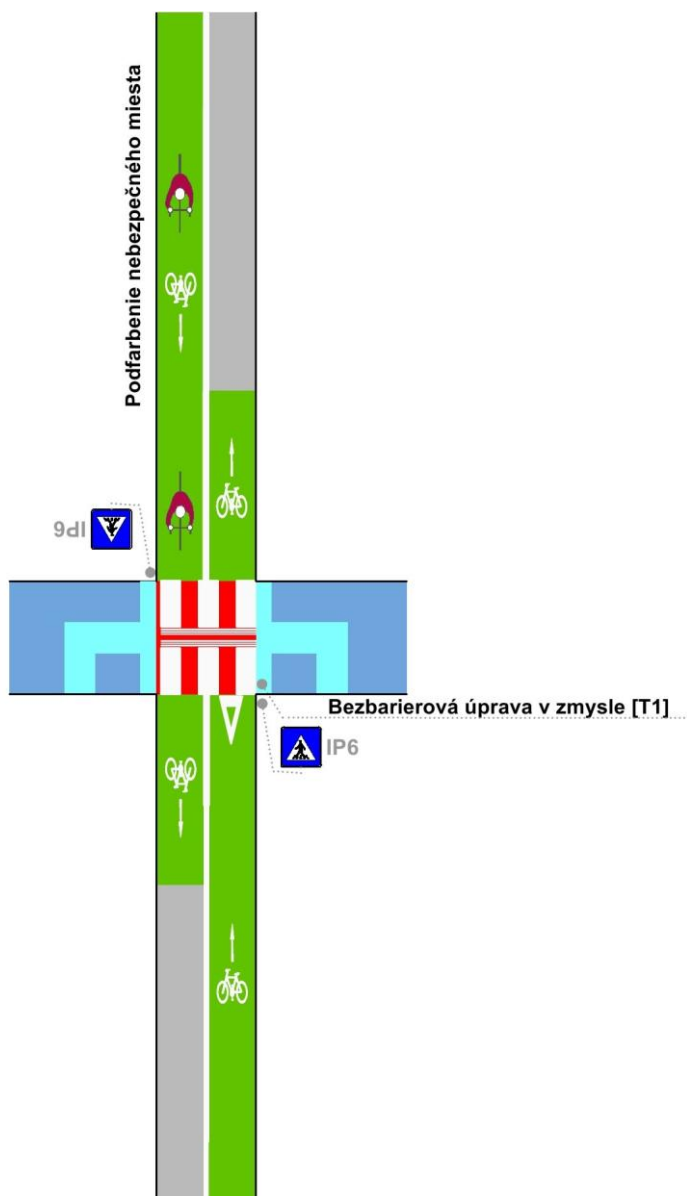
Obrázok 103 Križovanie pomocou priechodu pre chodcov s podfarbením a zároveň s podfarbením cyklistickej cestičky ako nebezpečného miesta
