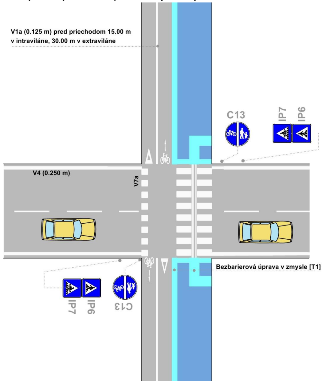
Obrázok 82 Nepodfarbený priechod pre cyklistov primknutý k priechodu pre chodcov
