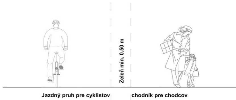
Obrázok 28 Oddelenie chodcov a cyklistov pomocou deliaceho pásu.
