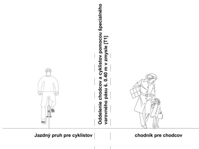
Obrázok 26 Oddelenie chodcov a cyklistov
