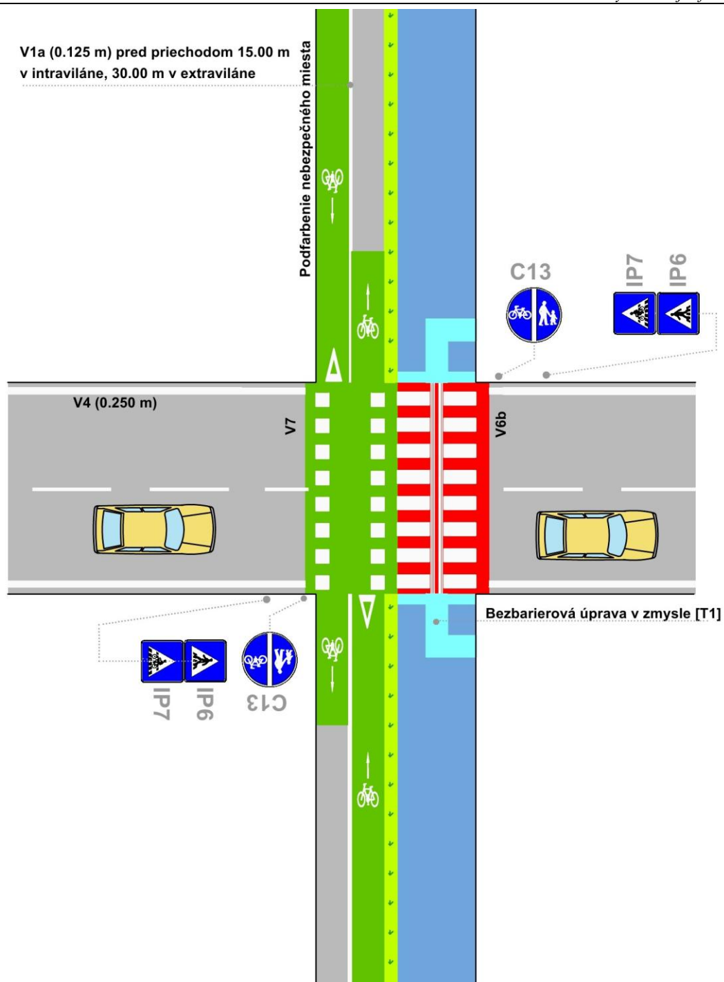
Obrázok 85 Podfarbený priechod pre cyklistov vedľa priechodu pre chodcov
