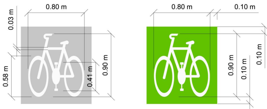
Obrázok 73 Rozmery piktogramu
