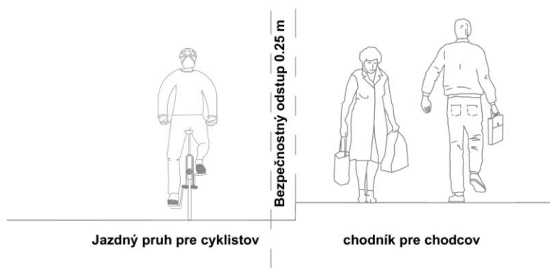
Obrázok 29 Oddelenie chodcov a cyklistov pomocou zvýšeného obrubníku
