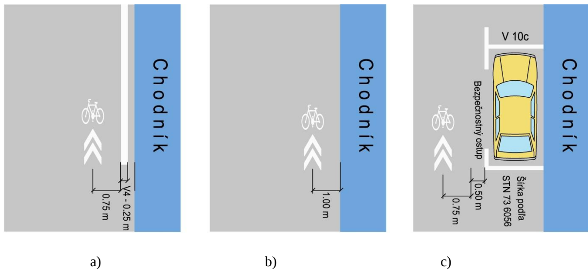
Obrázok 31 a), b), c) Vedenie cyklistického koridoru po PK
